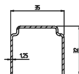
Art.-Nº. V 104 I_x = 2,4 \text{ cm}^4
