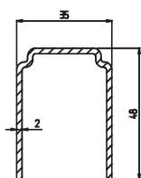
Art.-Nº. V 106 I_x = 5,3 \text{ cm}^4
