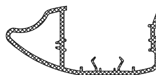
Interlock Art.-Nº. 9C57
